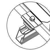
DETALLE E Abrazadera Universal (Modo Remate)
