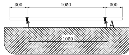
VISTA LATERAL
