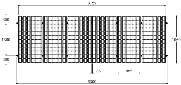
VISTA PLANTA
