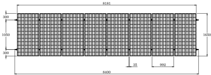
VISTA PLANTA
