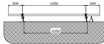
VISTA LATERAL
