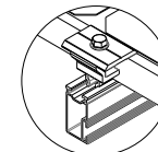
DETALLE B Abrazadera Universal (Modo Remate)
